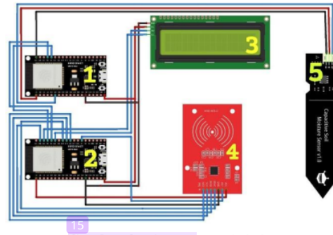
Gambar 3. Diagram Pengkabelan
