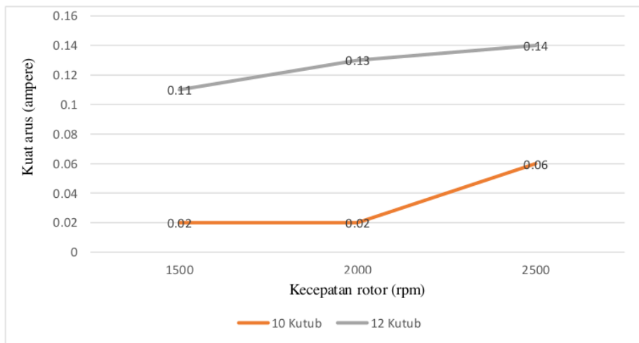
Gambar 22. Grafik Hasil Perbandingan Ampere pada 10 Dan 12 Kutub Kumparan Dengan 1500 rpm, 2000 rpm dan 2500 rpm
