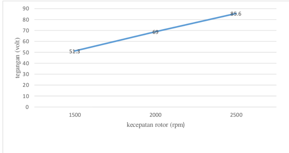
Gambar 16. Grafik Hasil Pengukuran Voltase Generator Dengan 12 Kutub kumparan
