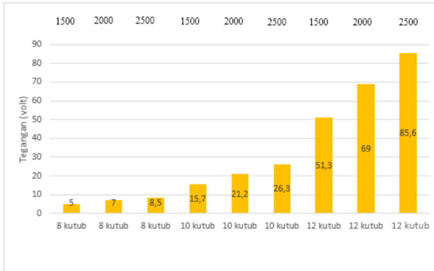
Gambar 23. Grafik Hasil Perbandingan voltase pada 8, 10, 12 Kutub Kumparan Dengan 1500 rpm, 2000 rpm dan 2500 rpm
