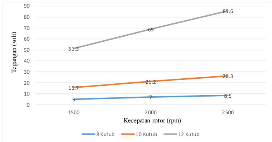
Gambar 21. Grafik Hasil Perbandingan voltase pada 8, 10, 12 Kutub Kumparan Dengan 1500 rpm, 2000 rpm Dan 2500 rpm
