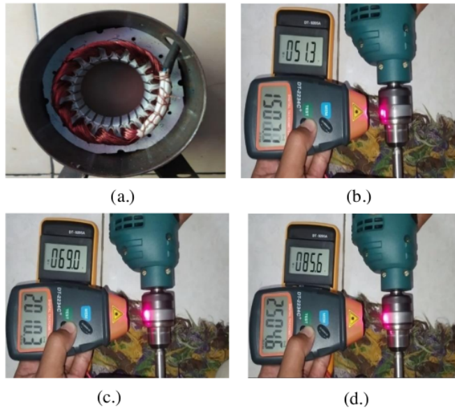
Gambar 13. Stator dengan 12 kutub kumparan b,c dan d hasil dari pengukuran voltase generator
