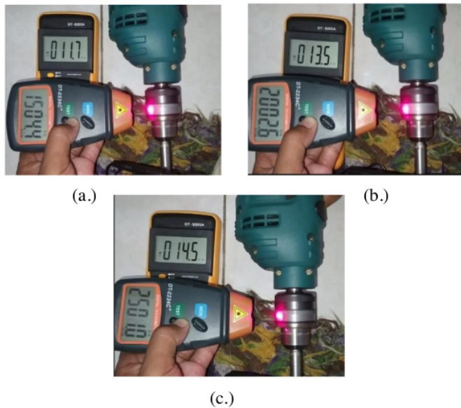
Gambar 14. Gambar a, b dan c hasil dari pengukuran ampere generator
