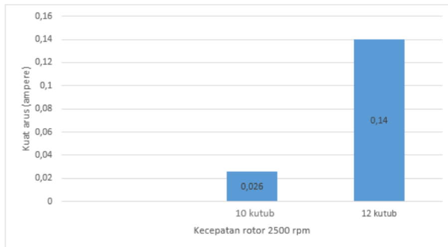
Gambar 26. Grafik Hasil Perbandingan Ampere Pada 10, dan 12 Kutub Kumaran Dengan Kecepatan 2500 rpm
