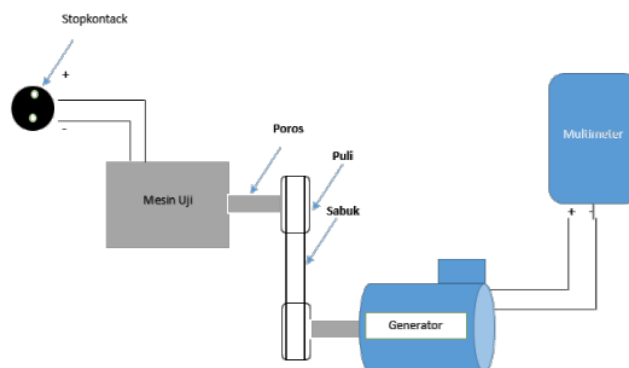
Gambar 5. Instalasi Pengujian Tanpa beban
