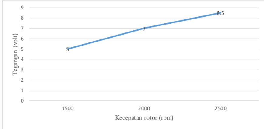
Gambar 8. Grafik Hasil Pengukuran Voltase Generator Dengan 8 Kutub Kumbaran
