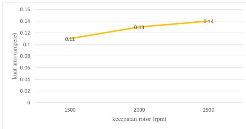
Gambar 15. Grafik Hasil Pengukuran Ampere Generator Dengan 12 Kutub kumparan
