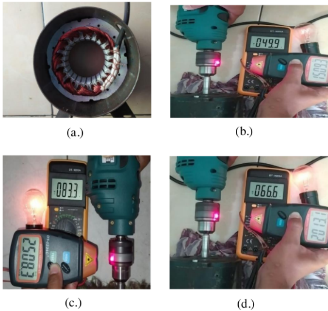
Gambar 17. Hasil Pengukuran Voltase Generator Dengan 12 Kutub kumparan dengan beban lampu 5 watt
