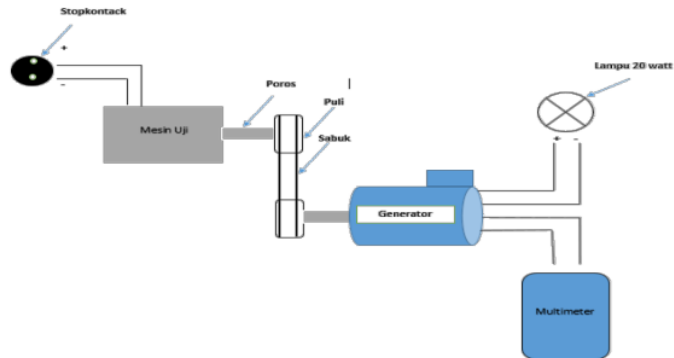
Gambar 6. Instalasi Pengujian Berbeban
