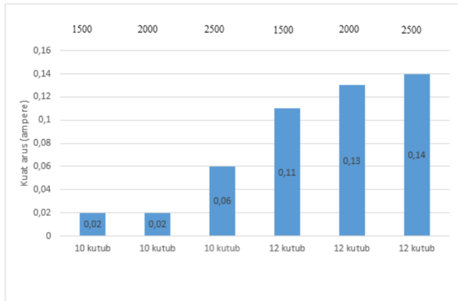
Gambar 24. Grafik Hasil Perbandingan Ampere pada 10 Dan 12 Kutub Kumbaran Dengan 1500 rpm, 2000 rpm dan 2500 rpm
