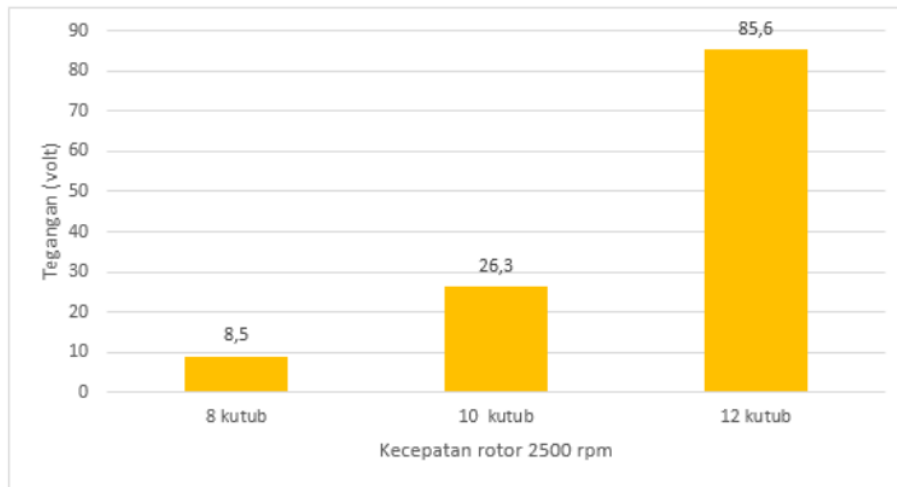
Gambar 25. Grafik Hasil Perbandingan Voltase Pada 8, 10, dan 12 Kutub Kumaran Dengan Kecepatan 2500 rpm
