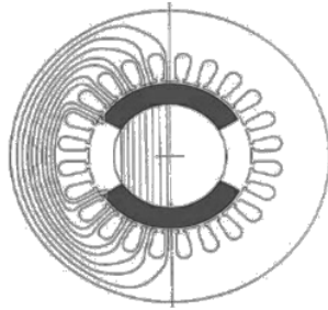
Gambar 3. Aliran fluks magnet pada desain generator
