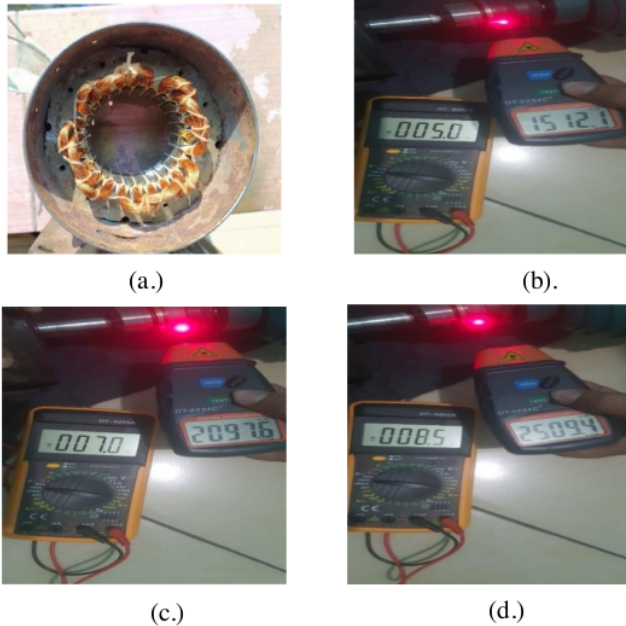
Gambar 7. a. Stator dengan 8 kutub kumbaran b,c dan d hasil dari pengukuran voltase generator.
