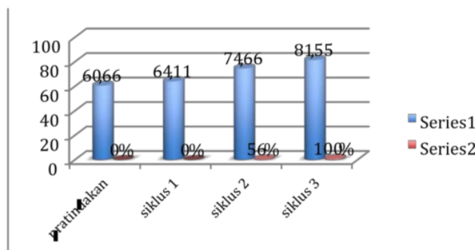
Gambar 1 Pratindak Siklus
