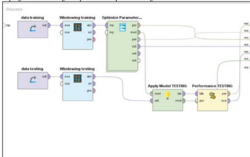
Gambar 1. Tahapan Implementasi Jaringan Syaraf Tiruan
