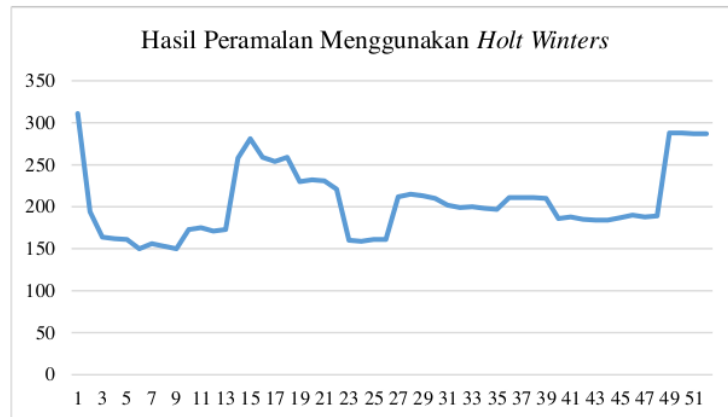
Gambar 5. Grafik Hasil Peramalan Menggunakan Metode Holt Winters
