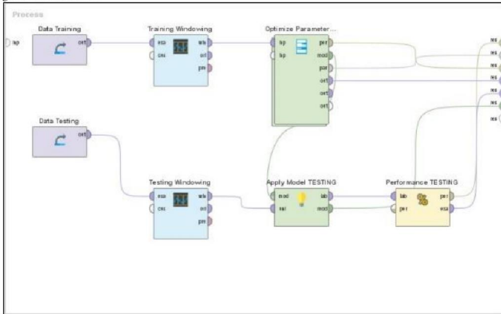
Gambar 2. Struktur Rancangan Artificial Neural Network Menggunakan Software Rapidminer .
