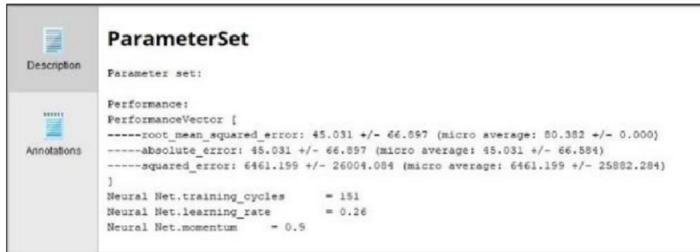
Gambar 5. ParameterSet Rapidminer
