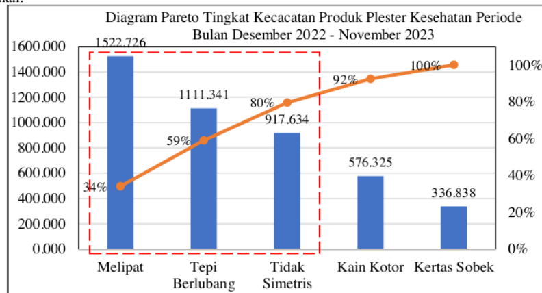
10 Gambar 2. Pareto Diagram Kecacatan Produk
