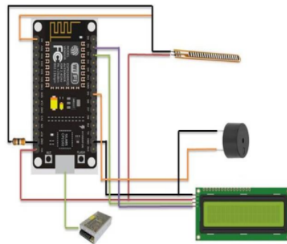
Gambar 3. Rangkaian alat koreksi postur berbasis NodeMCU
