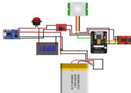
Gambar 3. Koneksi Alat
