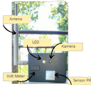
Gambar 5. Hasil Akhir Alat Sistem Pengawasan Rumah
