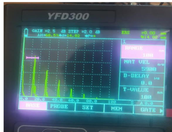
Gambar 17 Hasil Data Layar Pengujian Posisi 1 Pertama
