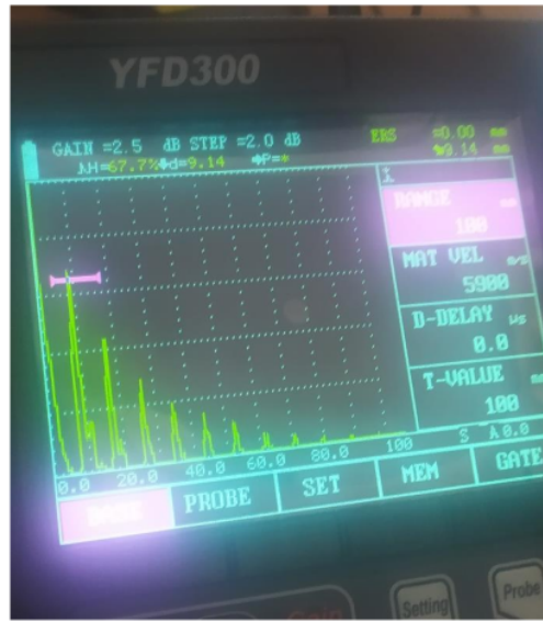
Gambar 33 Hasil Data Layar Pengujian Posisi Ketiga
