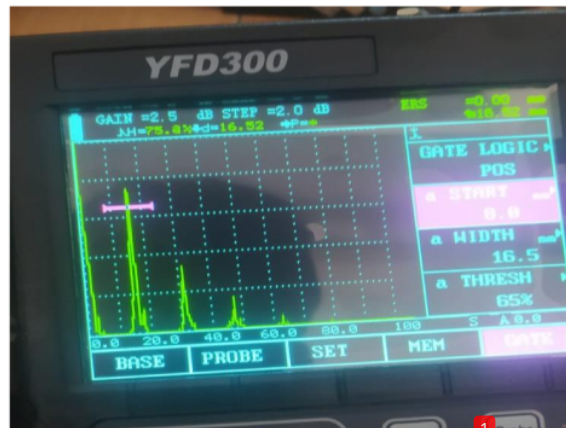
Gambar 13 Hasil Data Layar Pengujian Posisi Kedua
