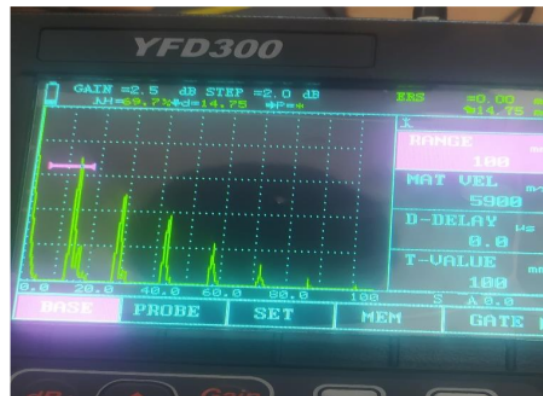
Gambar 21 Hasil Data Layar Pengujian Posisi Ketiga 1
