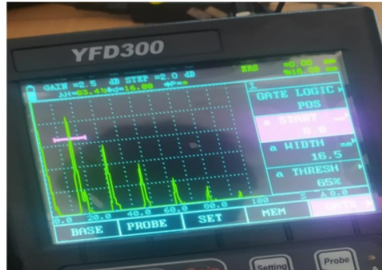
Gambar 15 Hasil Data Layar Pengujian Posisi Ketiga
