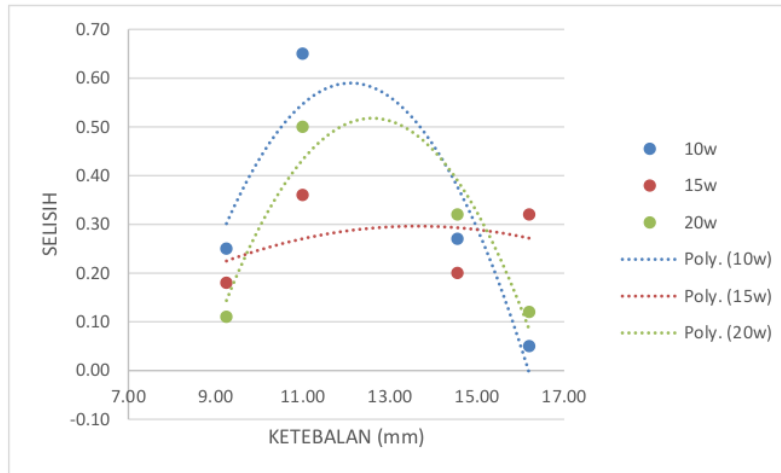
Gambar 34 Grafik Nilai Selisih Ketebalan Stabilisasi Kuplan
