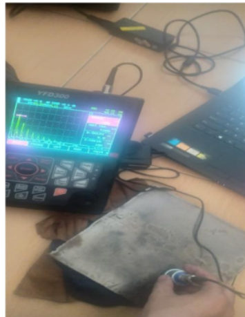
Gambar 32 Posisi Pengujian Ketiga
