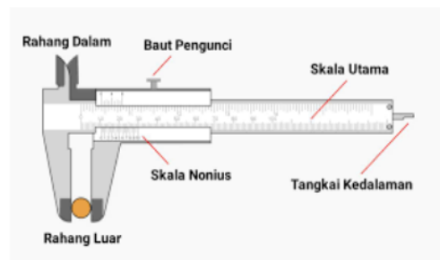
Gambar 7 Alat Ukur Jangka Sorong
