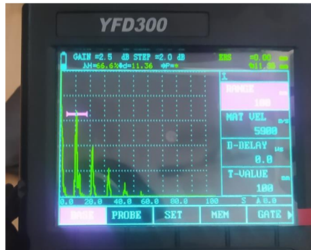
Gambar 25 Hasil Data Layar Pengujian Posisi 1 Kedua
