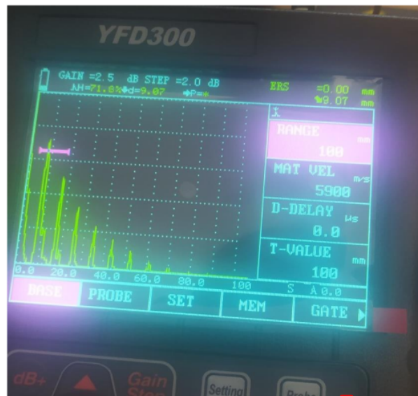
Gambar 31 Hasil Data Layar Pengujian Posisi Kedua
