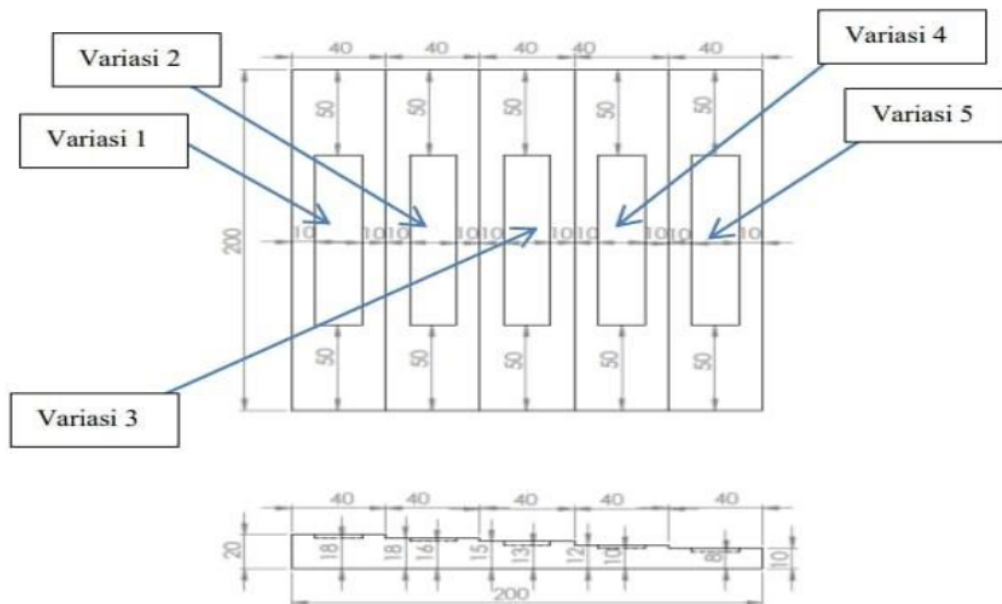
Gambar 9 Gambar Dan Rancang Ukuran Specimen
