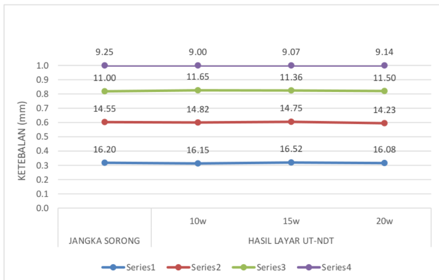
Gambar 35 Grafik Perbedaan Nilai Ketebalan Specimen Antara Pengujian Penggunaan Jangka Sorong Dan Alat Ultrasonik Testing
