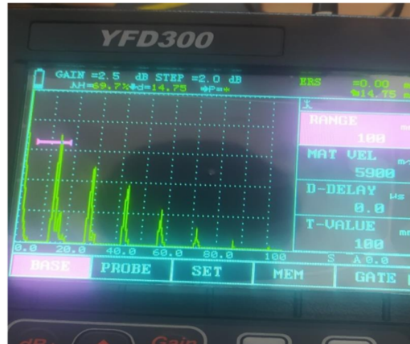
Gambar 19 Hasil Data Layar Pengujian Posisi Kedua
