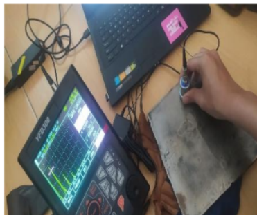
Gambar 12 Posisi Pengujian Kedua
