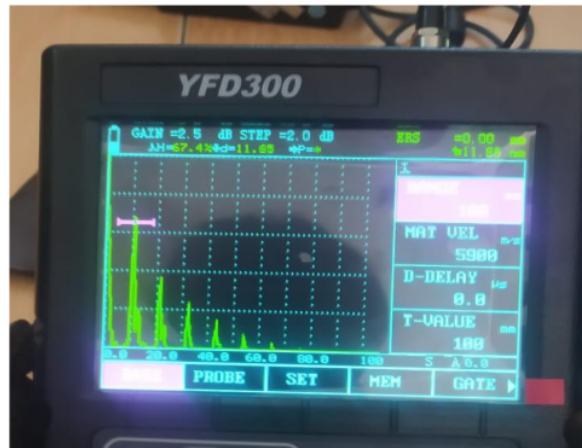
Gambar 23 Hasil Data Layar Pengujian Posisi 1 Pertama
