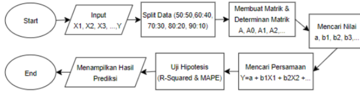
Gambar 4. Langkah-langkah Regresi
