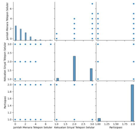
Gambar 2. Seaborn plot atau visualisasi data
