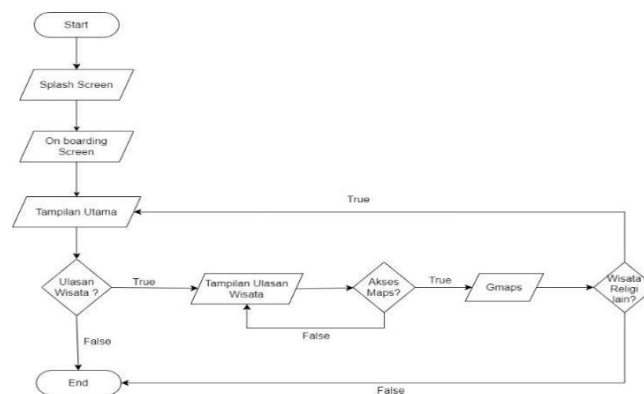
Gambar 2. Flowchart Aplikasi
