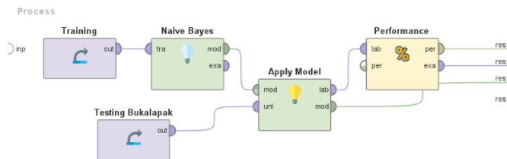
Gambar 3.6 Proses Klasifikasi Naïve Bayes
