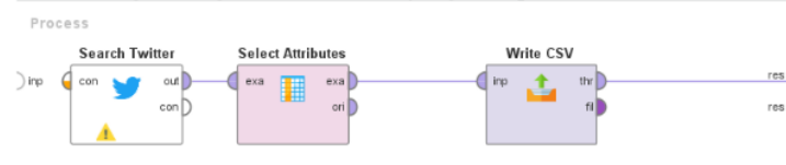
Gambar 3.1 Pengumpulan Data
