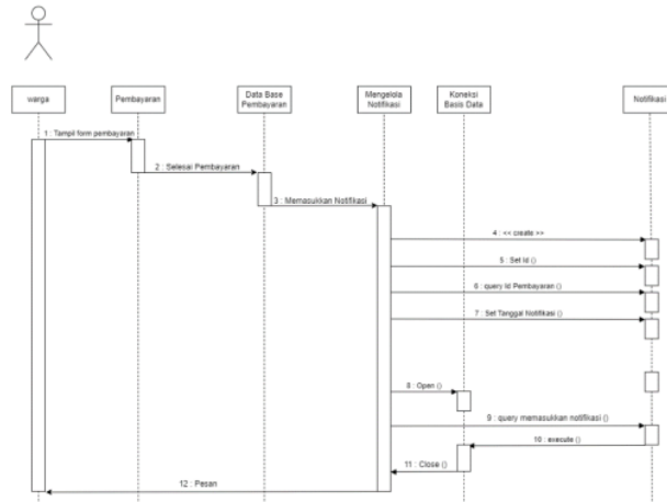
Gambar 9 Sequence diagram notifikasi
