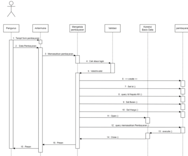
Gambar 8 Sequence diagram pembayaran
