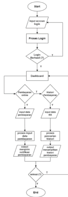
Gambar 3 Flowchart Pengguna
