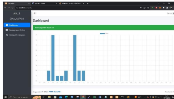
Gambar 13 tampilan warga
