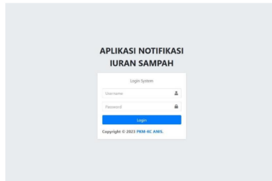
Gambar 11 Tampilan login
