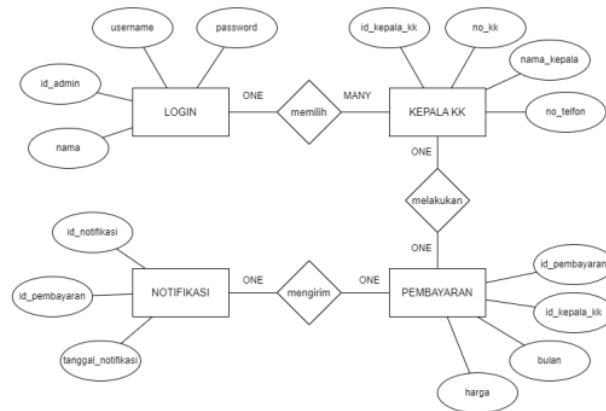
Gambar 10 ERD
