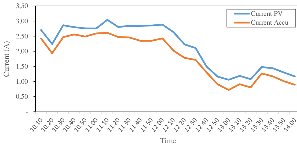
Gambar 6. Arus Panel Surya dan Aki
