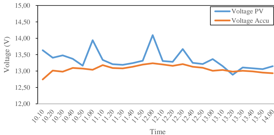
Gambar 5. Tegangan Panel Surya dan Aki
