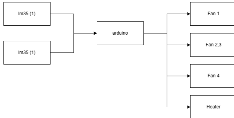
Gambar 3. Blok Diagram Sistem Kontrol
