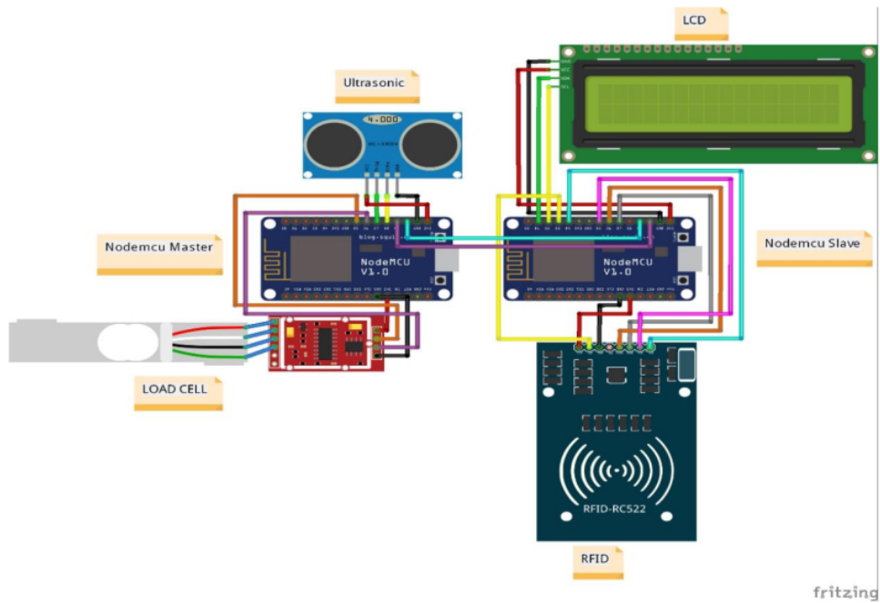
Gambar 1. Desain Pengkabelan
