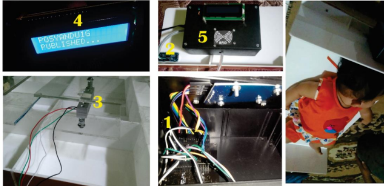
Gambar 5. Realisasi Alat
