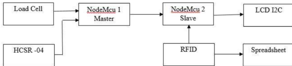
Gambar 4. Blok Diagram Sistem
