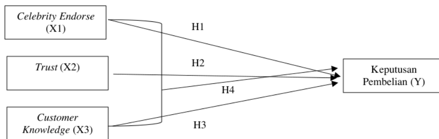
Gambar 2. Kerangka Konseptual
