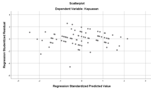
Gambar 3. Uji Heteroskedastisitas
