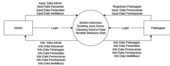
Gambar. 5. Diagram konteks
