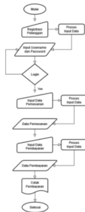
Gambar. 4. Flowchart pelanggan
