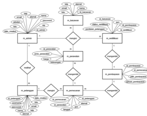
Gambar. 7. ERD sistem
