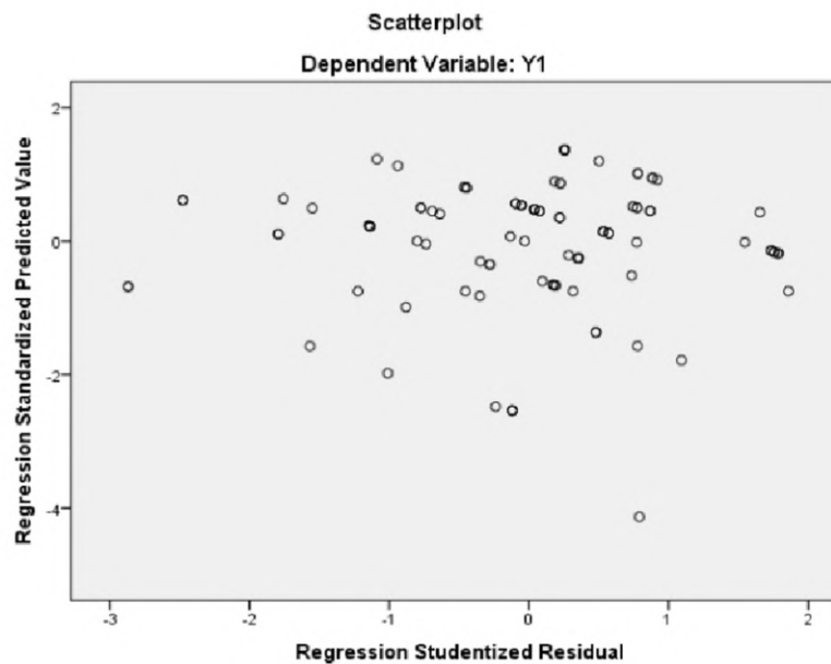
Gambar 2. Hasil Uji Heteroskedastistas Sumber: Hasil Olah Data, 2023
