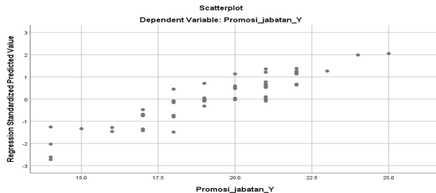
Gambar 1. Uji Heteroskedastisitas
