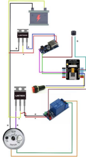
Picture 2. Rangkaian Keseluruhan Alat
