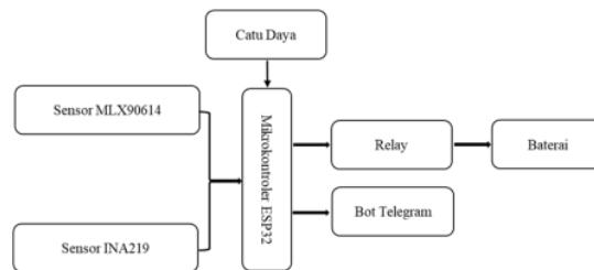
Gambar 6. Desain Perancangan Alat
