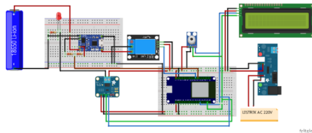
Gambar 8. Perancangan Hardware
