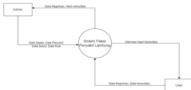
Gambar 3. Diagram Konteks
