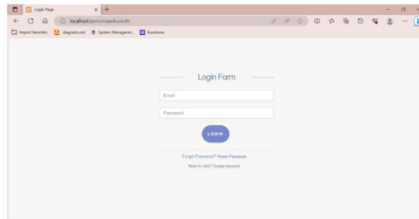
Gambar 8. Menu Login
