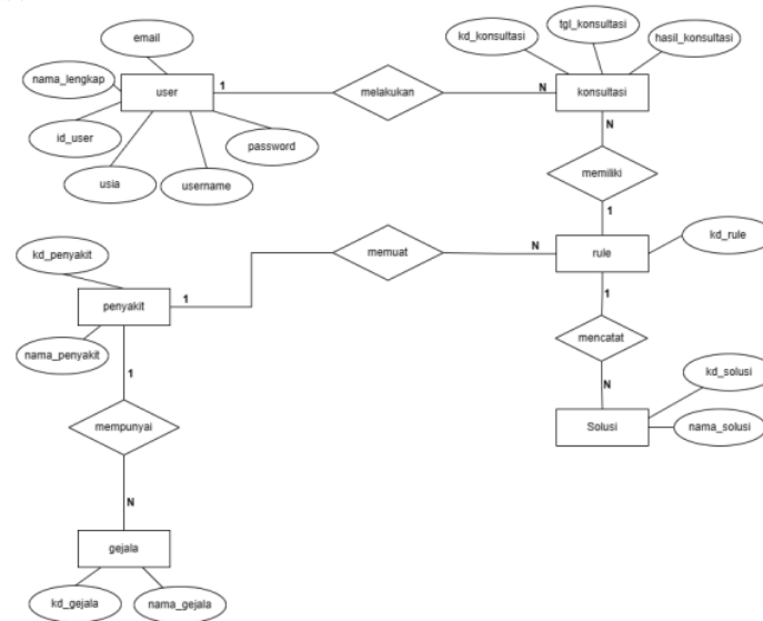
Gambar 4. ERD
