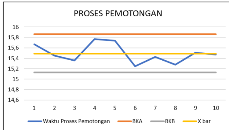
Gambar 2. Grafik uji keseragaman data pemotongan
