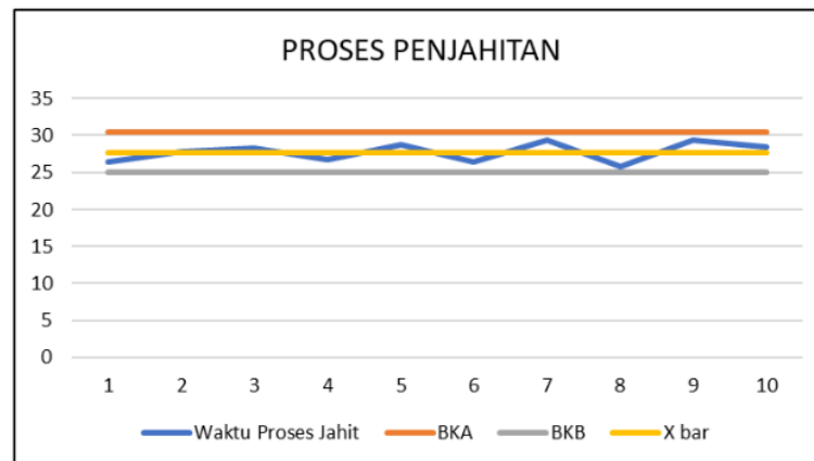
Gambar 3. Grafik uji keseragaman data penjahitan
