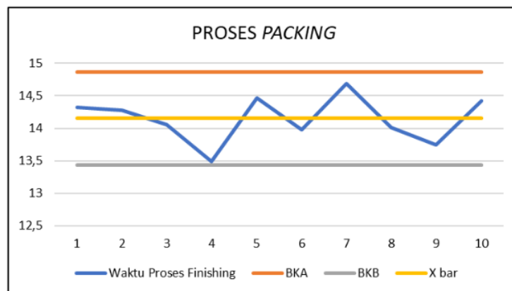
Gambar 6. Grafik Uji Keseragaman Data Packing
