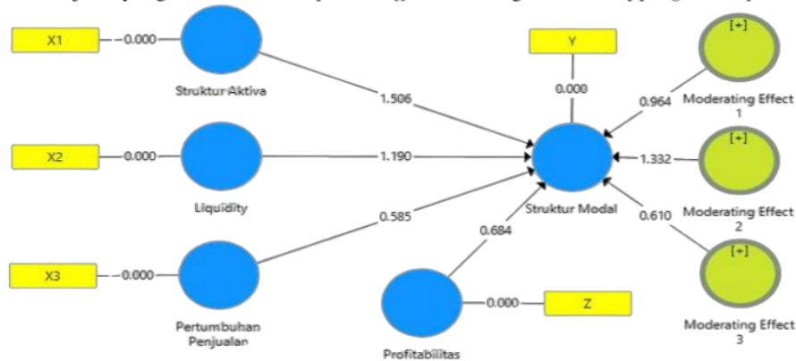
Gambar 2. Model Struktural Path Coefficients Dengan Bootstrapping Sumber : Output Smart PLS (2023)
