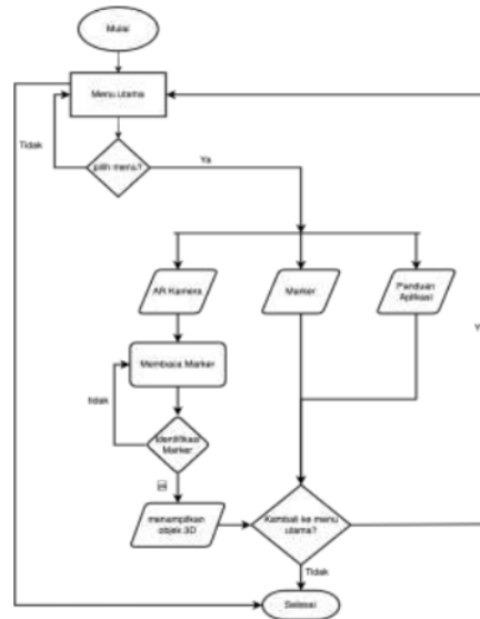
Gambar 5. Flowchart penggunaan aplikasi
