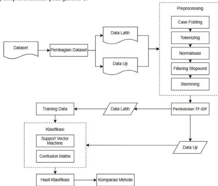
Gambar 2. Kerangka Alur Penelitian
