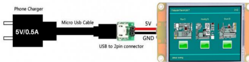
Gambar 5. Koneksi wiring Nexion HMI
