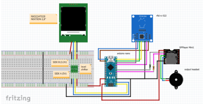
Gambar 9. Wiring keseluruhan alat
