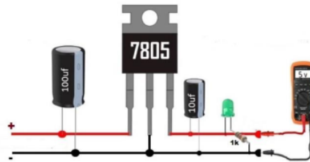
Gambar 10. Pengujian rangkaian regulator
