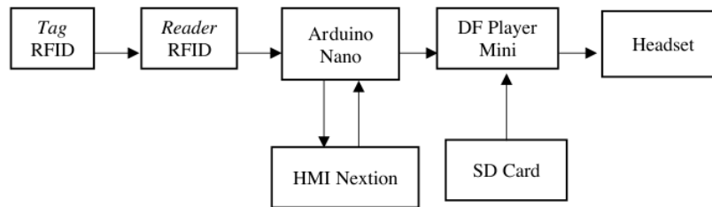
Gambar 1. Diagram Blok Sistem yang kami buat saat ini.
