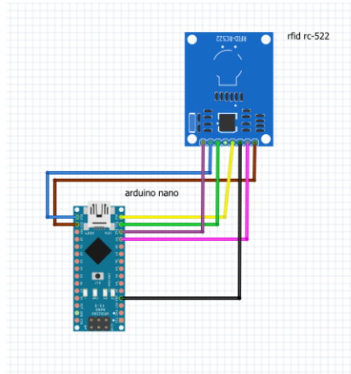
Gambar 6. Koneksi wiring RFID Reader MFRC522
