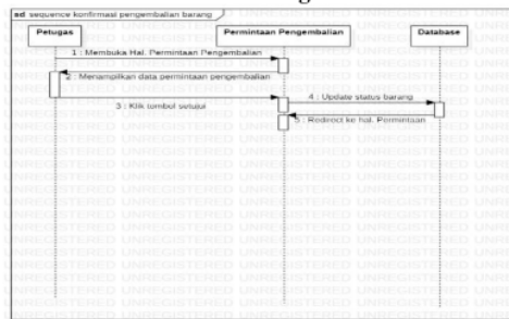
Gambar 11. Sequence Diagram Konfirmasi Pengembalian Barang
