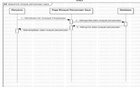
Gambar 13. Sequence Diagram Riwayat Penyewaan Pelanggan
