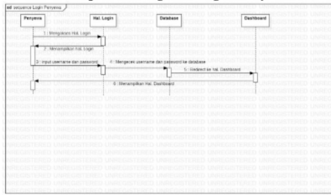
Gambar 7. Sequence Diagram Login Penyewa
