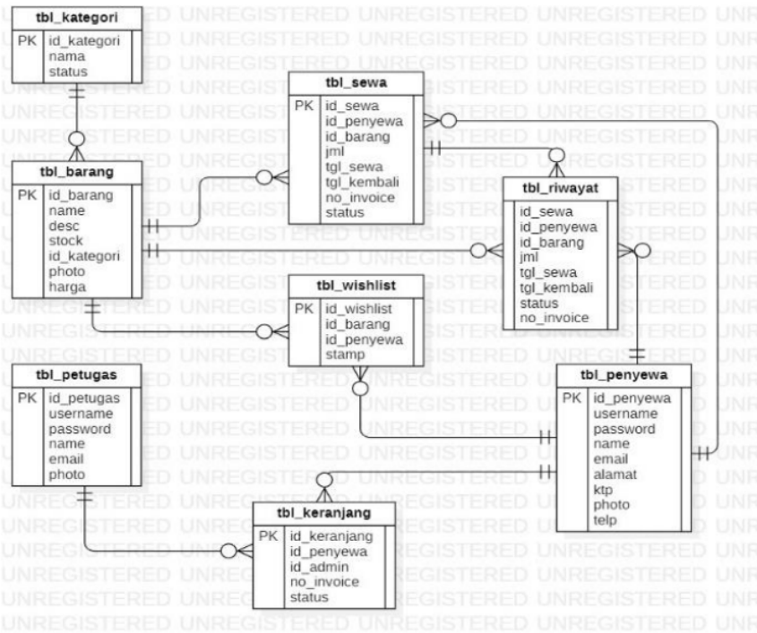
Gambar 22. ERD Sistem informasi penyewaan pada InOutdoors Rental
