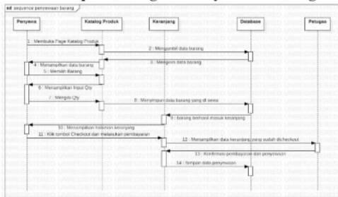
Gambar 8. Sequence Diagram Penyewaan Barang
