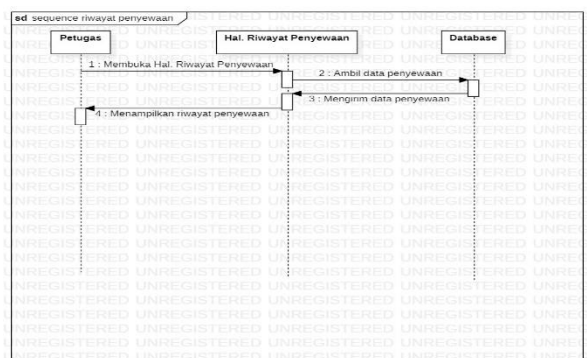
Gambar 12. Sequence Diagram Riwayat Penyewaan Petugas
