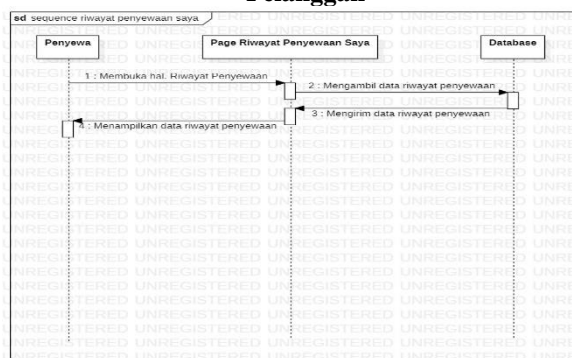
Gambar 13. Sequence Diagram Riwayat Penyewaan Pelanggan
