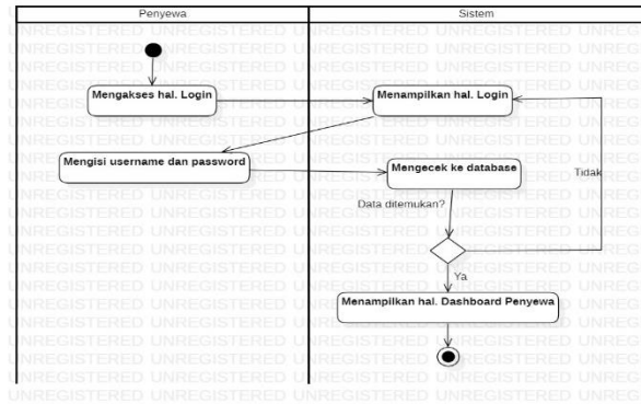
Gambar 15. Diagram Activity Login Penyewa
