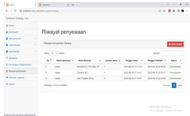
Gambar 30. Halaman Riwayat Penyewaan (Admin)
