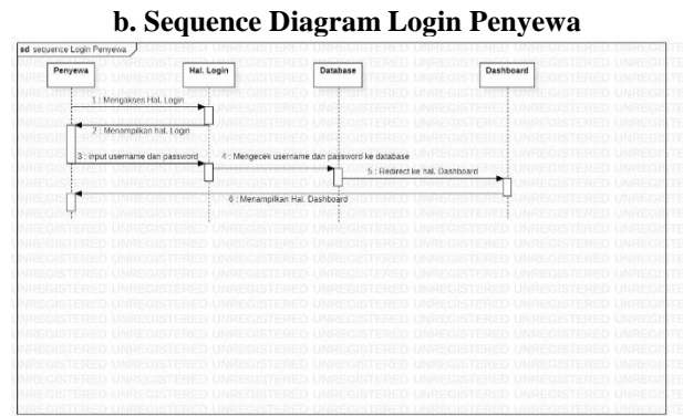
Gambar 7. Sequence Diagram Login Penyewa
