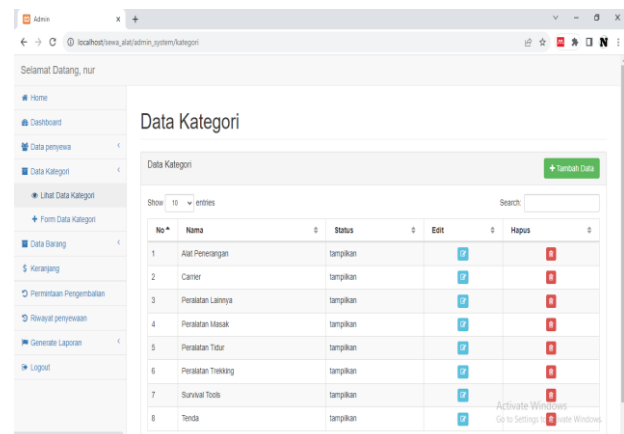
Gambar 26. Halaman Data Kategori (Admin)
