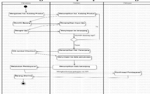
Gambar 16. Diagram Activity Penyewaan Barang
