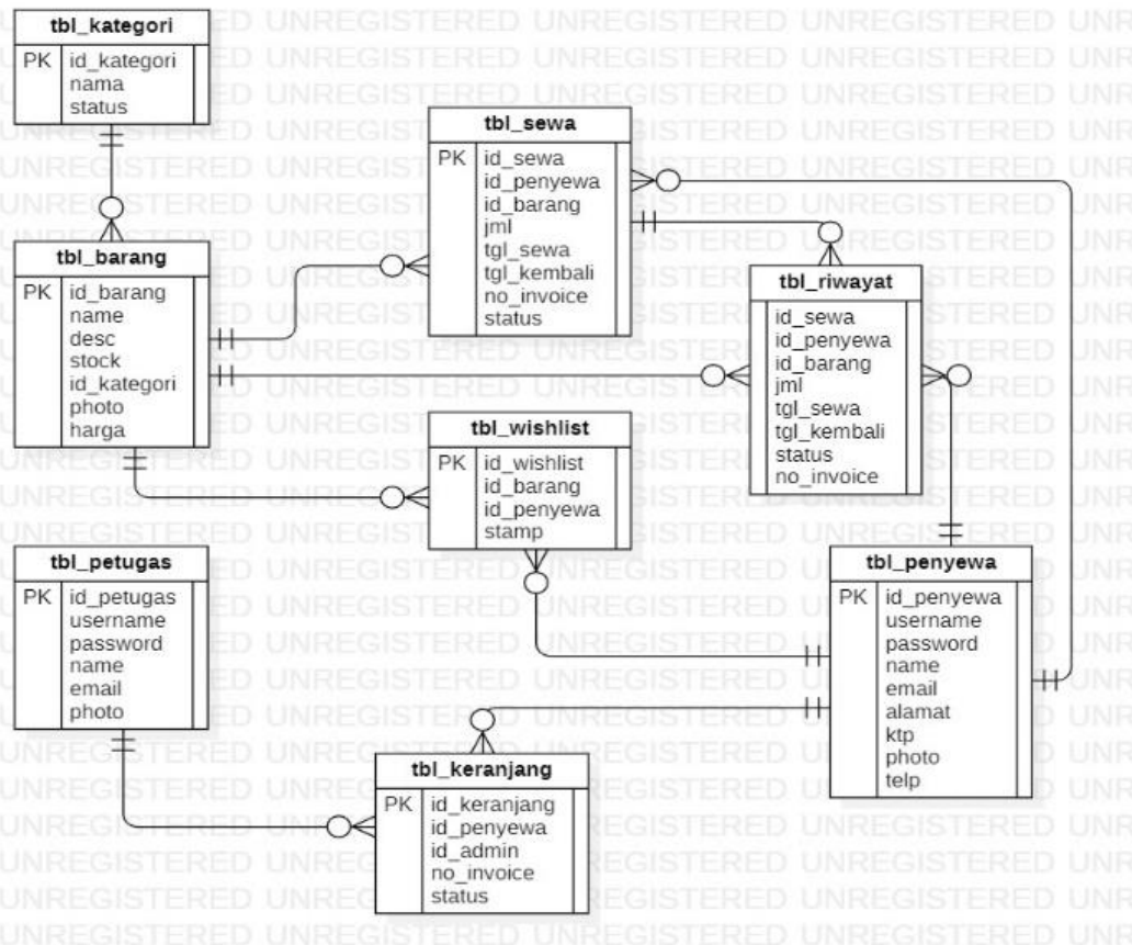
Gambar 22. ERD Sistem informasi penyewaan pada InOutdoors Rental
