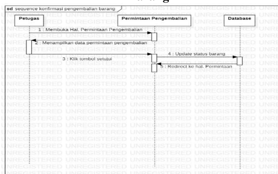
Gambar 11. Sequence Diagram Konfirmasi Pengembalian Barang
