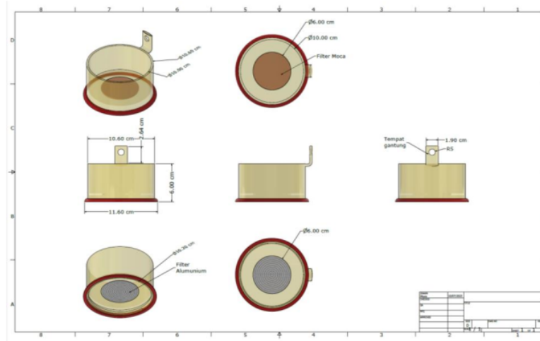
Gambar 5. Bagian Atas Bucket ENEMA Kopi
