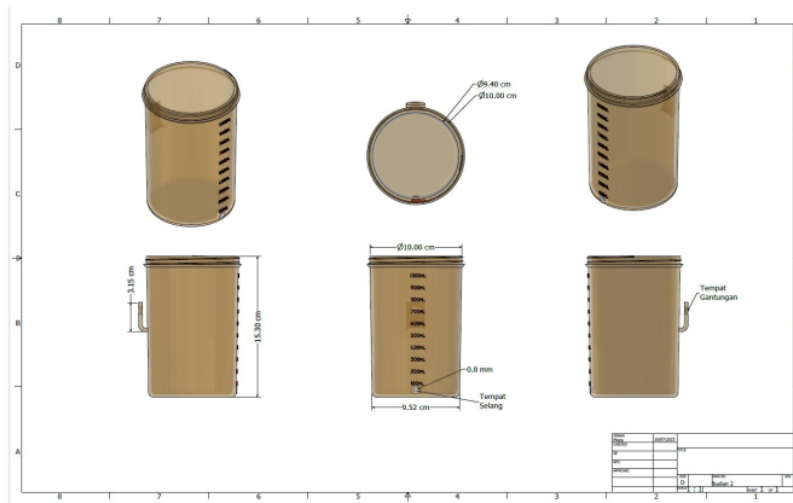
Gambar 4. Bagian Bawah Bucket ENEMA Kopi
