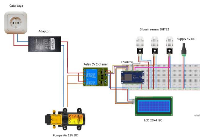
Gambar 3. Perancangan Perangkat Keras
