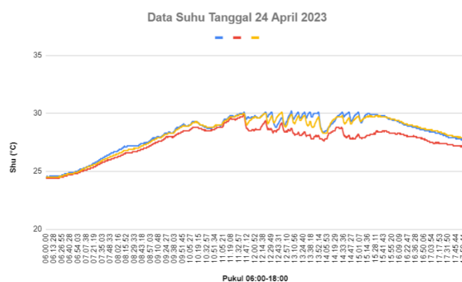
Gambar 6. Analisa fluktuasi suhu siang hari
