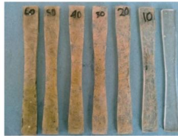
Gambar 4. Hasil Spesimen Uji Tarik
