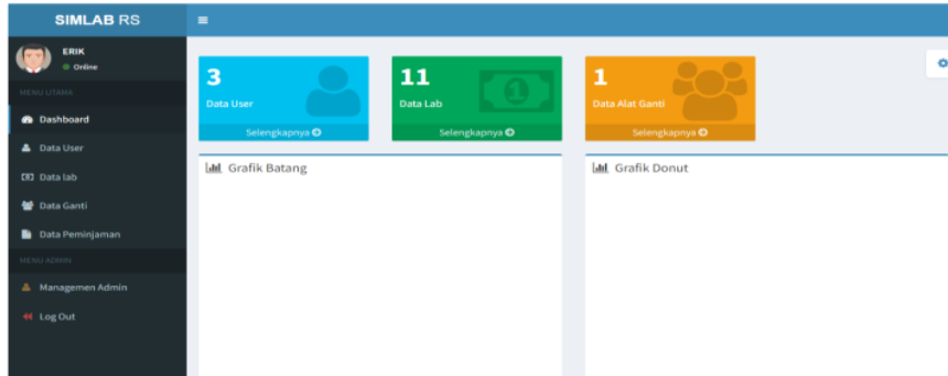
Gambar 8. Menu Utama
