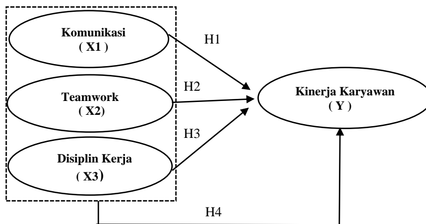
Gambar 1. Kerangka komseptual
