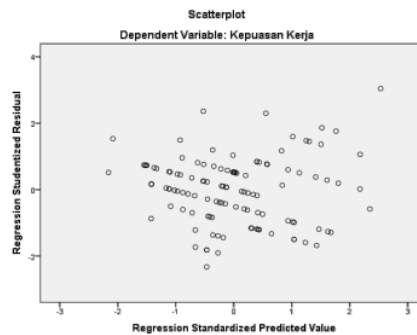
Gambar 3. Uji Heteroskedasitas
