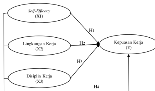
Gambar 1 : Kerangka Konseptual
