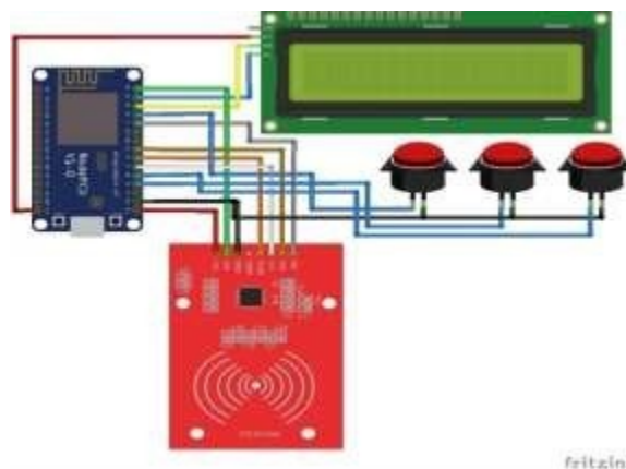
Gambar 3. Wiring Diagram Rangkaian Keseluruhan Alat
