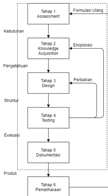
Gambar 2. Langkah-Langkah Metode ESDLC
