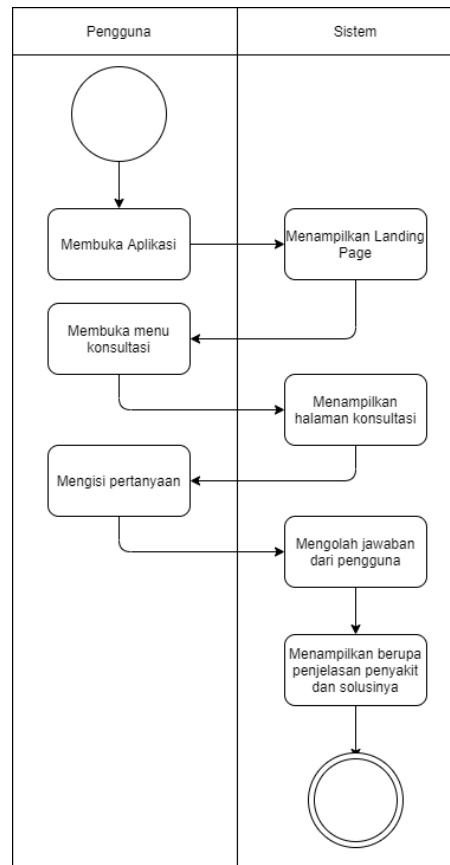
Gambar 3. Activity Diagram Aplikasi
