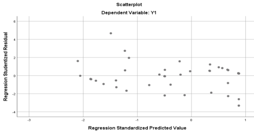
Gambar 2. Scatterplot Variabel Dependen : Minat Beli Konsumen Sumber : Data Diuji Menggunakan SPSS
