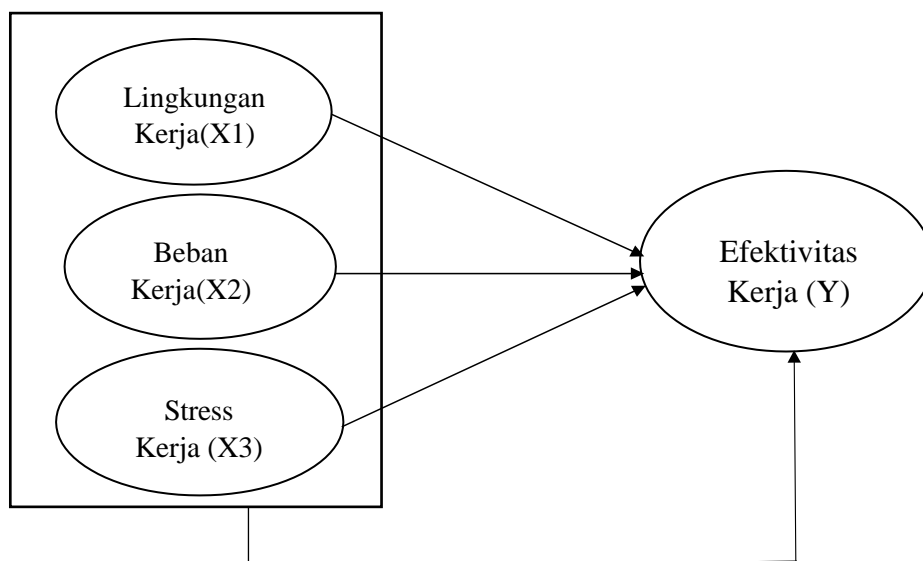
Gambar 1. Kerangka Konseptual
