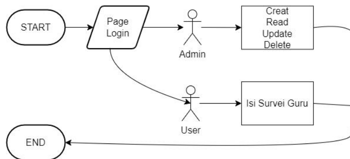
Gambar 1. Diagram Alur Perancangan Sistem Aplikasi
