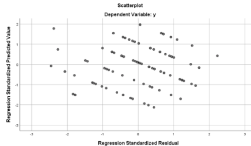
Gambar 2 Uji Heterokedastisitas
