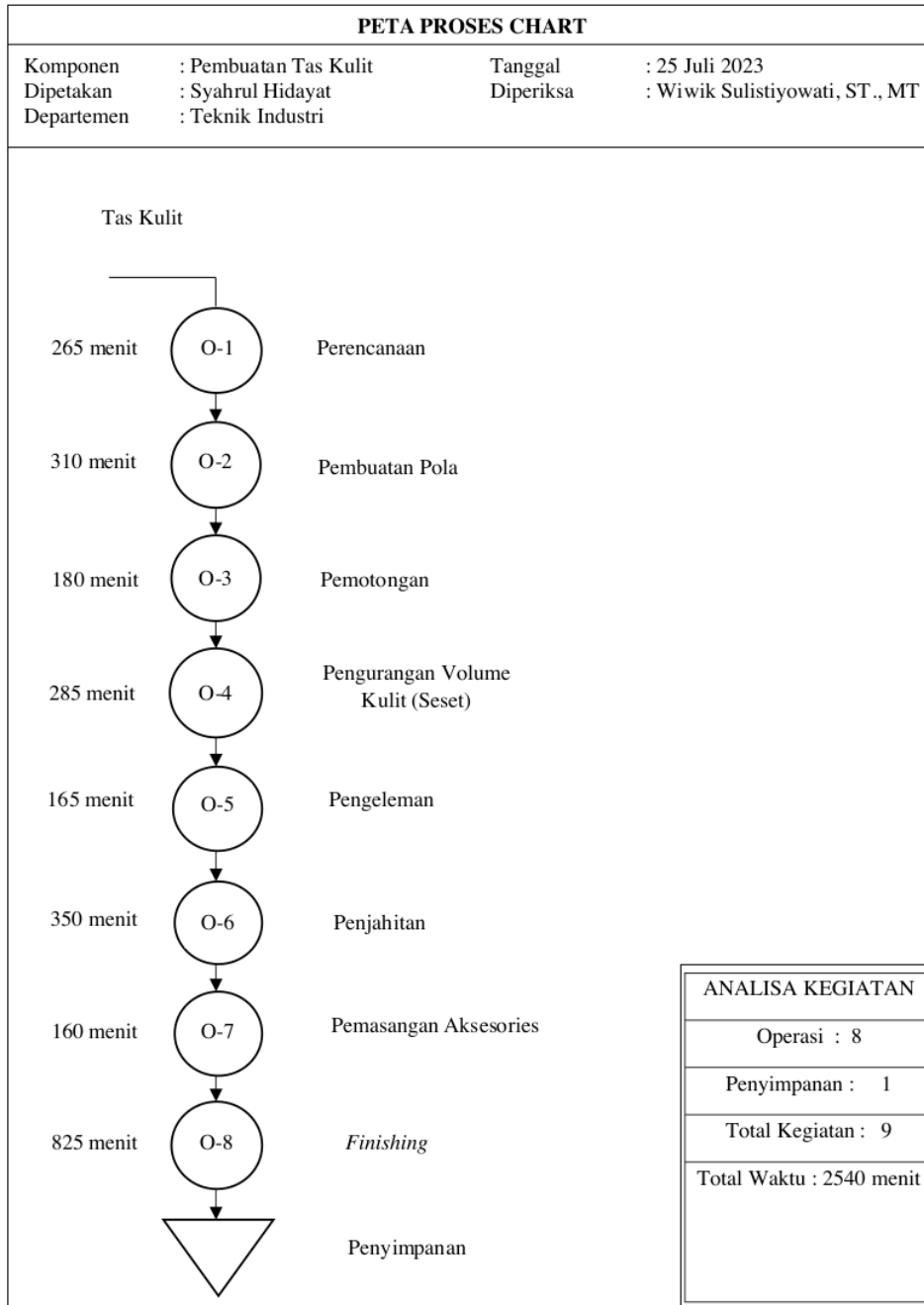
Gambar 2. Proses Produksi
