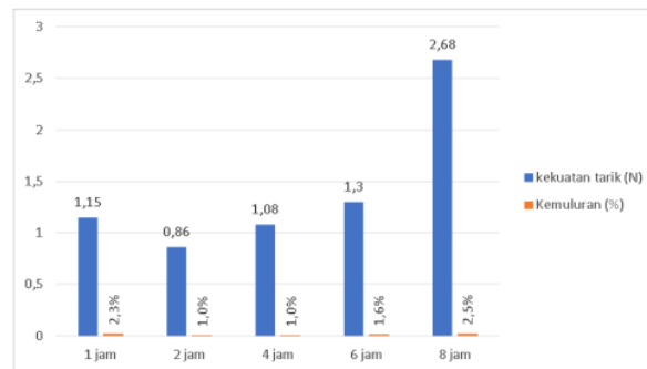
Gambar 6. Grafik uji Tarik serat
