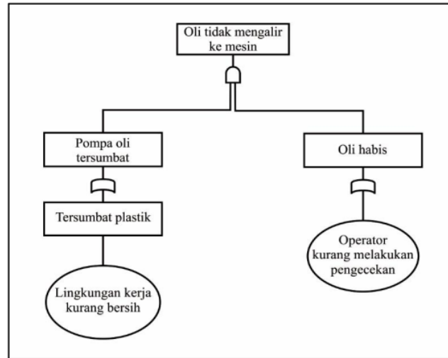
Gambar 4. FTA Oli Tidak Mengalir Ke Mesin
