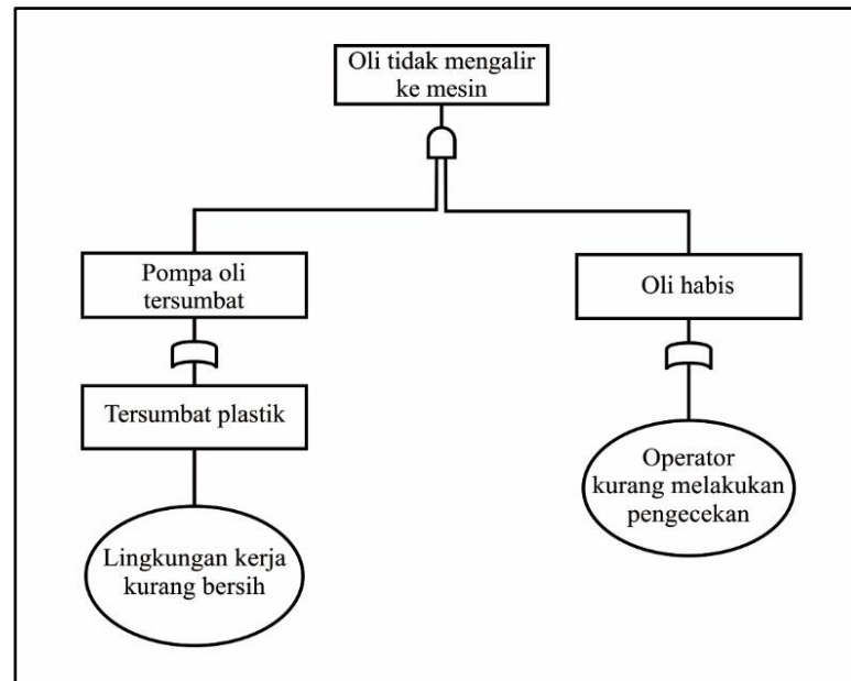
Gambar 4. FTA Oli Tidak Mengalir Ke Mesin
