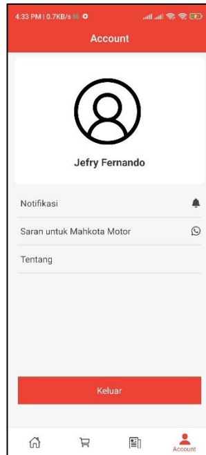
Gambar 15. Halaman Akun
