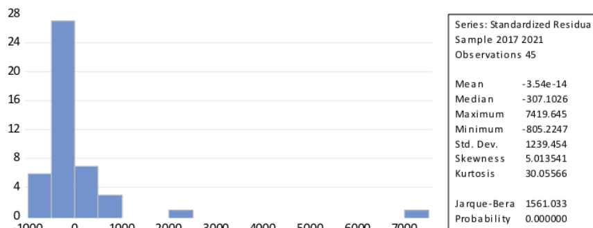
Gambar 3 Uji Normalitas
