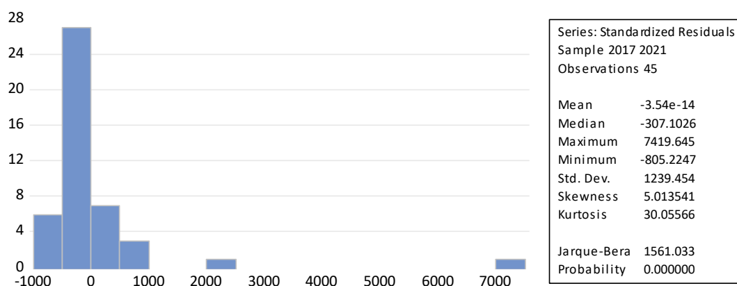
Gambar 3. Uji Normalitas
