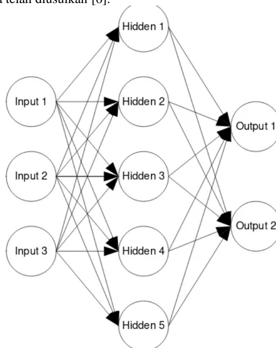
Gambar 1. Arsitektur Neural Network
